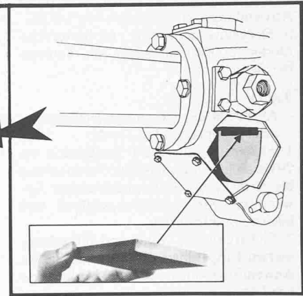
Eine Schnittansicht eines Teils der ausfahrbaren Lagerplatte eines «RAM»-Raupenbohrers zeigt eine rechteckige Platte aus KS Aramid. Das verschleissfesteste Material bildet die Lagerfläche für den Arm
