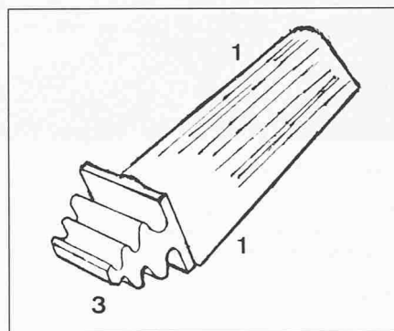
Bild 27. Unterschiedlich zu behandelnde Zonen an Turbinen und Kompressoren-Schaukeln. 1: eigentliche Arbeitsflächen der Schaufeln; 3: Wurzelnende der Schaufel (sogenannter «Tannenbaum»).
