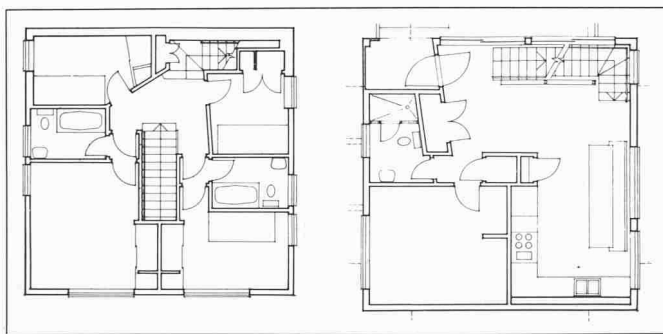
Eingangsgeschoss/Schlafgeschoss Brant Johnson House. Wohnungsgrundriss
