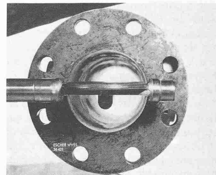
Bild 1. Modell einer Schwenklappe zur Messung der Druckverluste und der Geschwindigkeitsverteilung
