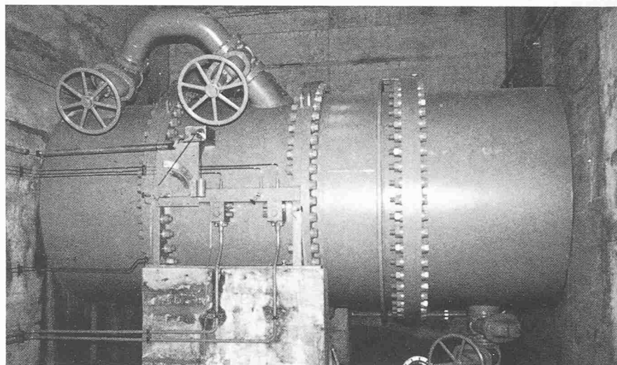
Bild 2. Drosselklappe Nr. 4 in eingebautem Zustand
