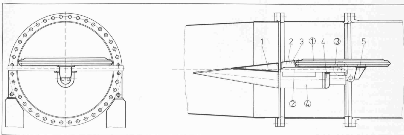
Bild 3. Schwenklappe. 1 Drehteller, 2 Querträger, 3 Abstützung, 4 Servomotor, 1 + 5 Strömungskörper
