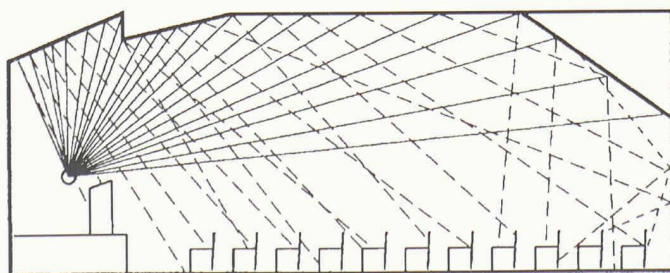
1 Anwendung geometrischer Akustik in einem kleinen Vortragssaal [1]
