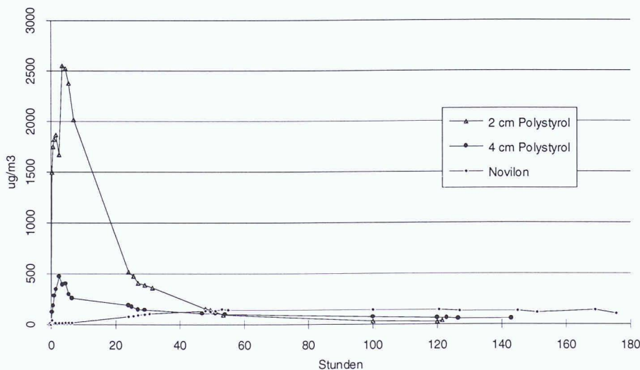
Bild 7. Einfluss des Abdeckmaterials auf die gemessenen Konzentrationen von Toluol in der Prüfkammer
