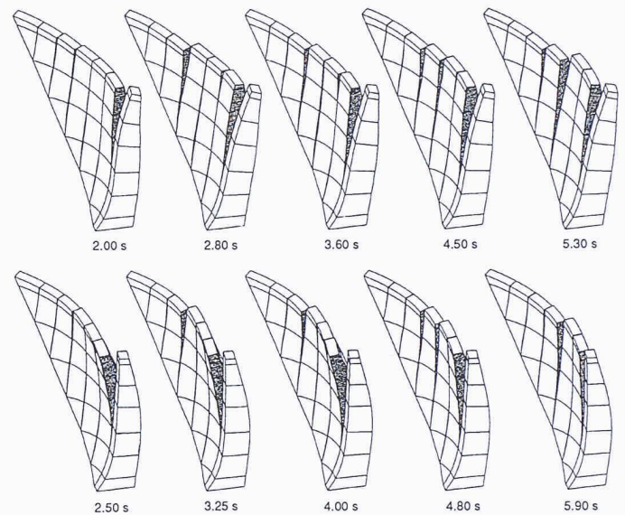
Bild 7. Bogenstaumauer mit geöffneten Blockfugen zu verschiedenen Zeiten während eines Erdbebens (nichtlineares Computermodell)
