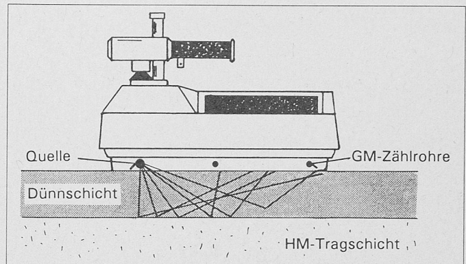
Rückstreuverfahren
