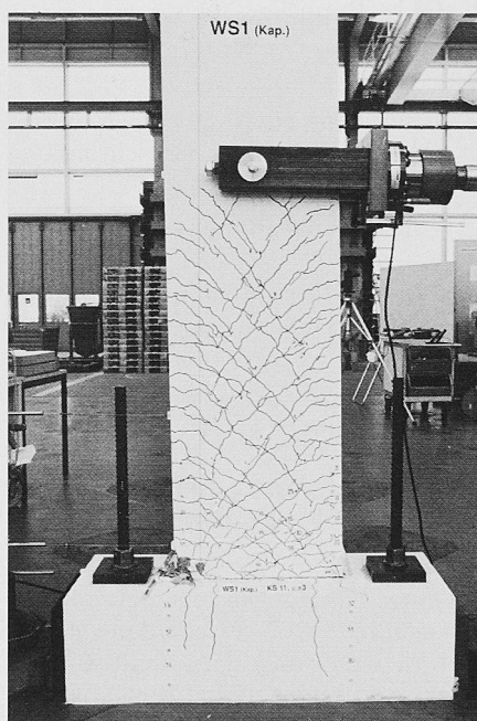
Bild 4. Statisch-zyklisch geprüfte Stahlbetontragwände im Massstab 1:3: konventionell bemessene Wand WS2 mit vorzeitigem Schubbruch (links); kapazitätsbemessene Wand WS1 mit duktilerem Verhalten (rechts)
