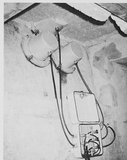
Bild 10. Überführung «du Milieu»: Verankerungshauben und elektrische Anschlüsse zur periodischen Überwachung der Spannglieder
