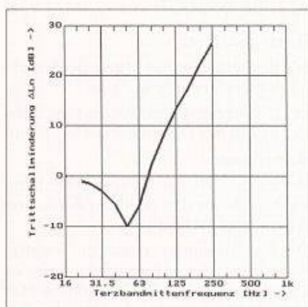
Darstellung der nach Beziehung (2) errechneten Trittschallminderung \Delta L_w des Unterlagsbodens (Der Verlustfaktor des Dämmmaterials wurde zu d = 0,10 angenommen)
