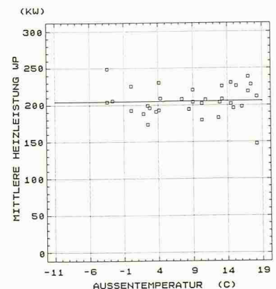
Heizleistung der Waermepumpe, Messdaten 1984-1987
