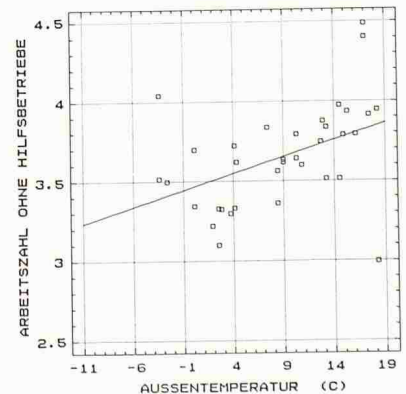
Arbeitszahl der Waermepumpe, Messdaten 1984-1987
