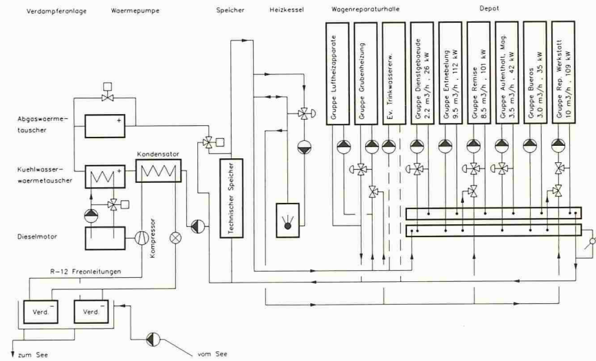
Prinzipschema der Anlage: Dieselmotorwärmepumpe mit Seewasser als Wärmequelle, bivalent parallel (-2 °C), Heizleistung 251.5 kW (64/50 °C, 4/2 °C), Leistungsziffer 3.14, Heizziffer 1.74
