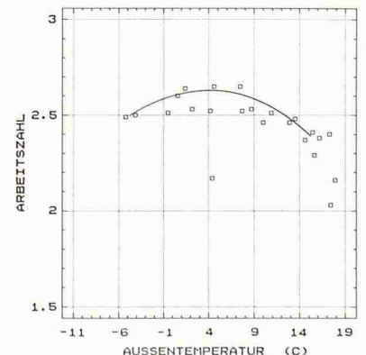
Arbeitszahl der Wärmepumpe, Messdaten 1984-1986
