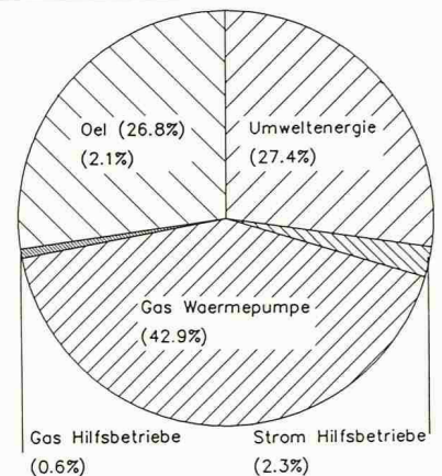
Energie-Einsatz 1984-1985
