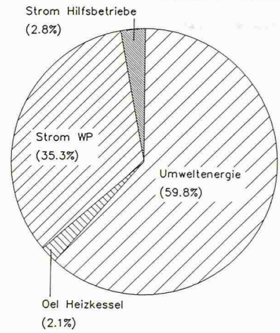
Energie-Einsatz 1984-1985 (kWh)
