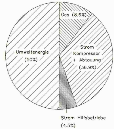
Energie-Einsatz 1986-1987
