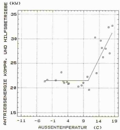
Elektrische Leistungsaufnahme Kompressor und Hilfsbetr., Messdaten 1985-1987
