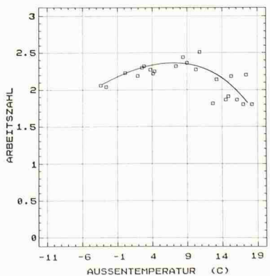
Arbeitszahl der Wärmepumpe, Messdaten 1985-1987
