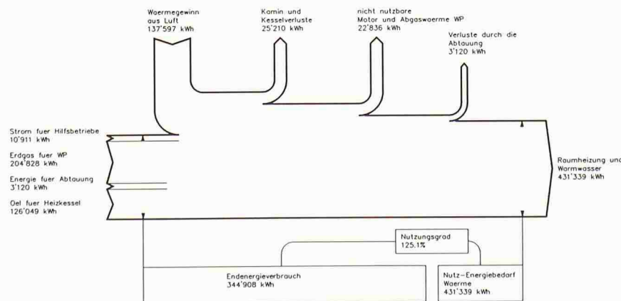
Energie-Flussdiagramm 1984-1985
