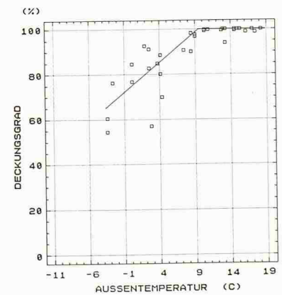
Anteil Waermelieferung der WP am Gesamtwärmebedarf, Messdaten 1984-1987
