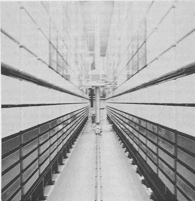
Bild 12. Vollautomatische, unbemannte Regalbediengeräte werden nicht nur für Paletten mit bis zu 40 m Höhe eingesetzt, sondern auch Behälter und Tablare lassen sich zuverlässig ein- und auslagern
