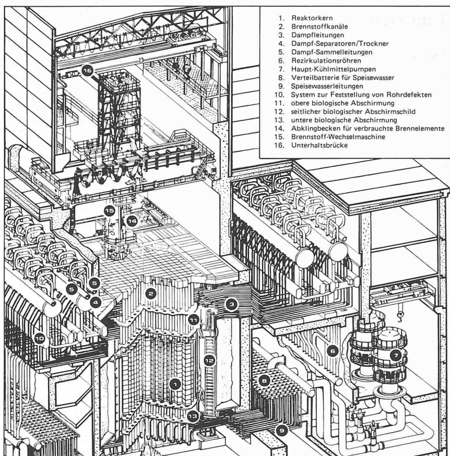
Bild 1. Schema des graphitmoderierten Leichtwasserreaktors, Typ RBMK (Bild IAE/SVA)
