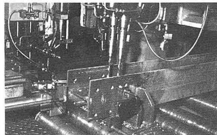
Bild 6. Auf der Bohrstrasse erhält ein Walzprofil die nötigen Schraubenlöcher
