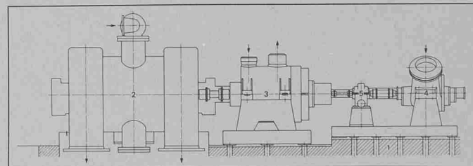
Mit der Modalanalyse untersuchte Maschinengruppe. Dampfturbine 2, Kesselspeisepumpe 3, Zubringerpumpe 4
