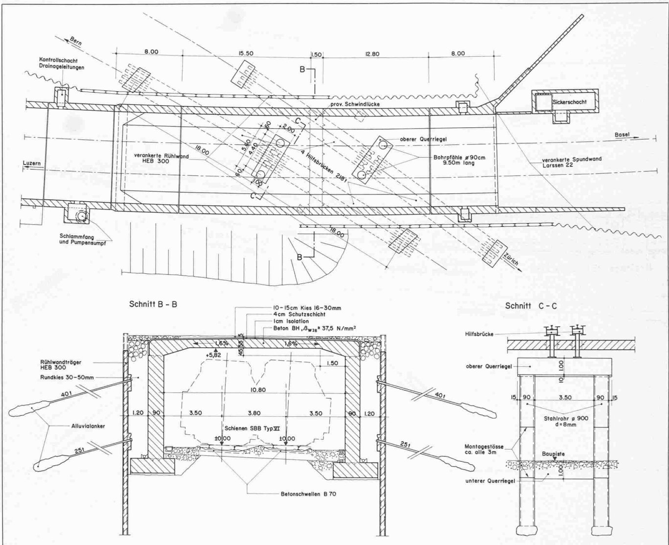
Bild 8. Überwerfungsbauwerk
