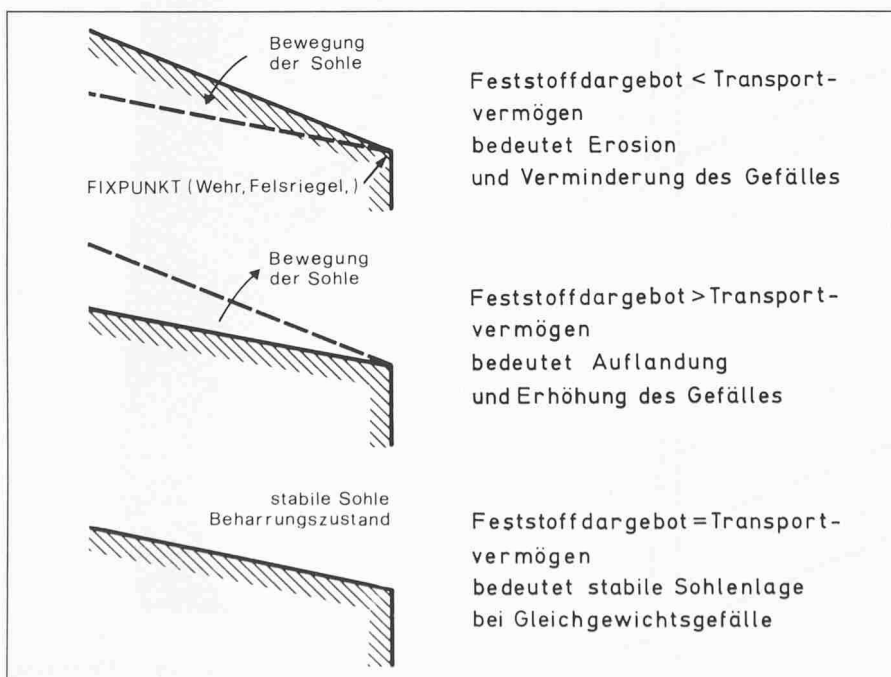
Bild 1. Drei schematische Längsschnitte eines Flusslaufs. Entwicklung des Sohlengefälles bei Erosion (oben) und bei Auflandung (Mitte). Beharrungszustand zwischen Feststoffdargebot und Transportvermögen (unten)
