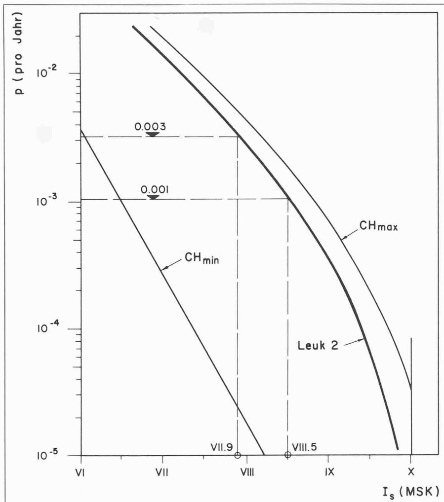
Bild 10. Risikobeziehung für den Standort der Antenne 2 in Leuk. Für die Standortintensität I_s können die zugehörigen Eintretenswahrscheinlichkeiten abgelesen werden. Zudem wird das Risiko in Leuk mit dem an extremen Standorten in der Schweiz verglichen ( CH_{max} , CH_{min} )
