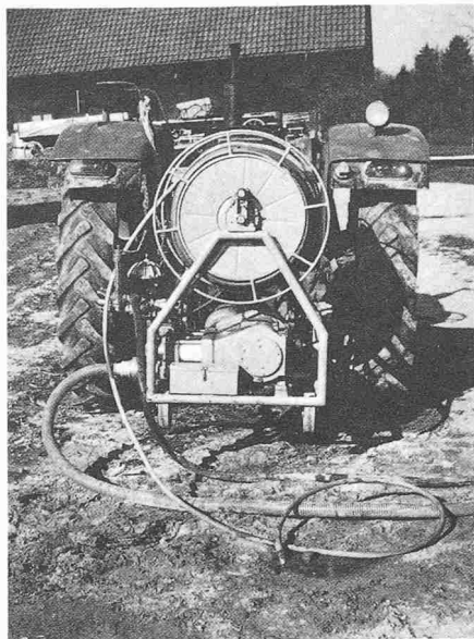
Bild 2. Angebautes Dränpülgerät «Fricke» am Dreipunktgestänge des Traktors
