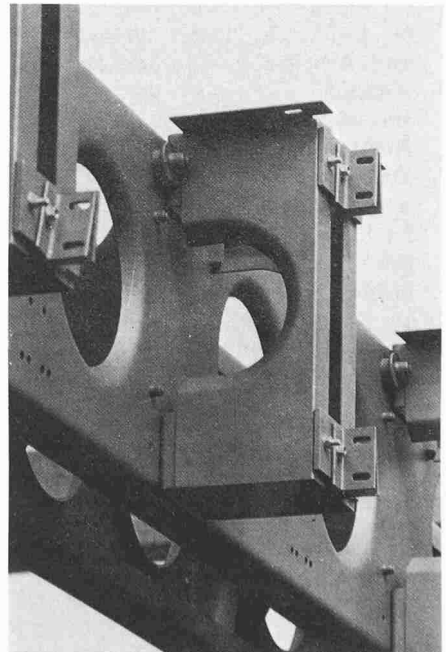
Detail Fassadenkonsole
