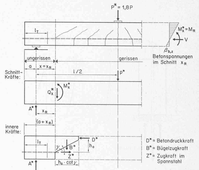
Bild 3. Auflagerbereich im Bruchzustand
