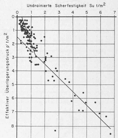
Bild 2. Drehflügelversuche in der Seekreide am Bielensee
