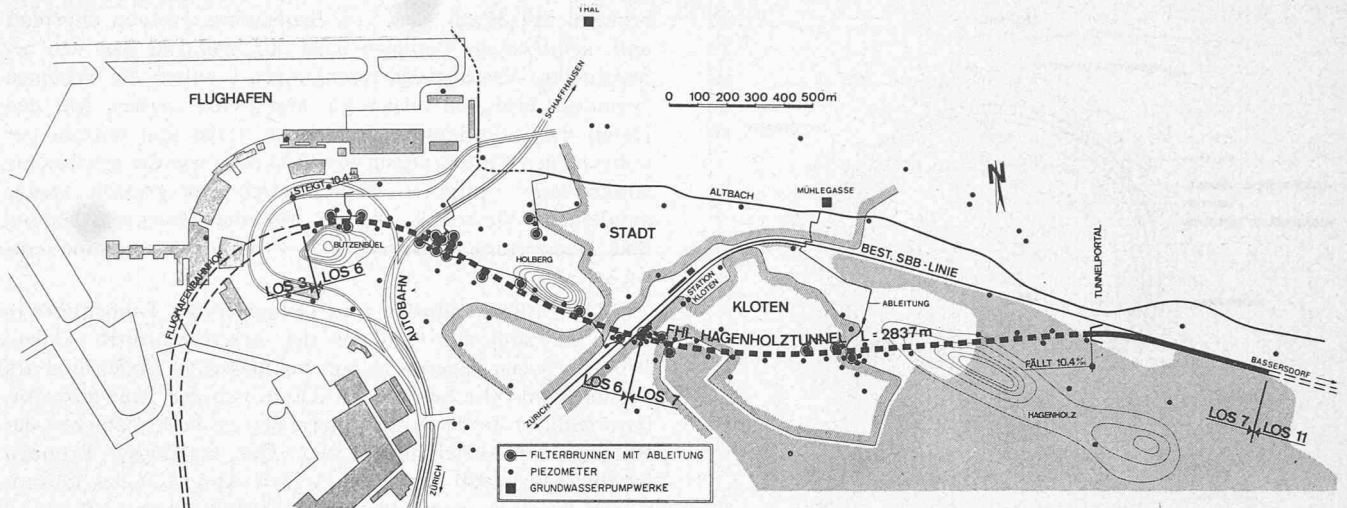
Bild 1. Situation mit Filterbrunnen und Piezometern für die Grundwasserabsenkung
