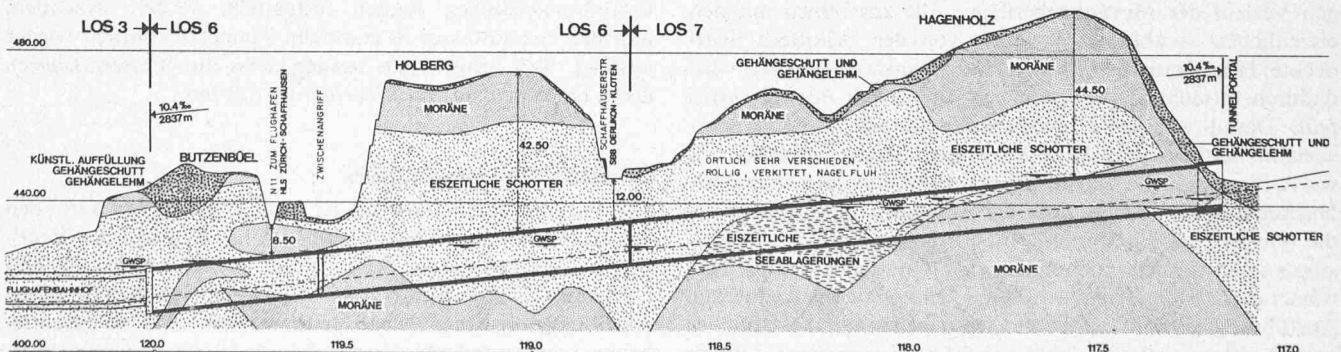
Bild 2. Geologisches Längensprofil
