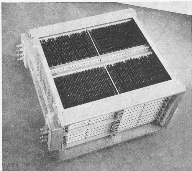
Bild 18. Bremswiderstand
