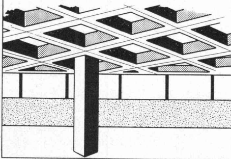
Kassetten- und Rippendecken-Schalkörper Verdrängungskörper und Schalelemente Bauwerks-Einstiegsöffnungen
