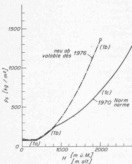
Bild 1. Neu vorgeschlagene (strichpunktierte gezeichnete Kurve) und bisher gültige (fest ausgezeichnete Kurve) Schneelast p_s als Funktion der Höhe H in m ü. M.
