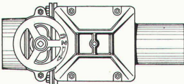
Triplex Doppel-Rückstauverschluss für durchgehende Rohrleitungen
