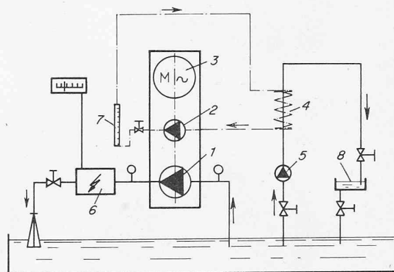
Bild 4. Versuchsanordnung schematisch
