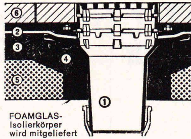
Dachterrasse, einteilig
