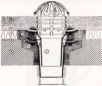
Kiesschüttdach, 2teilig
