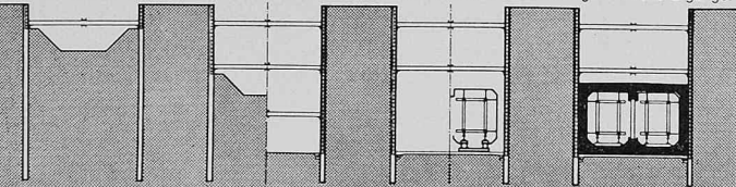
Bild 8. Ablauf der Baugruben- und Tunnelherstellung bei verschiedenen Verbaumethoden, entnommen aus [9]
