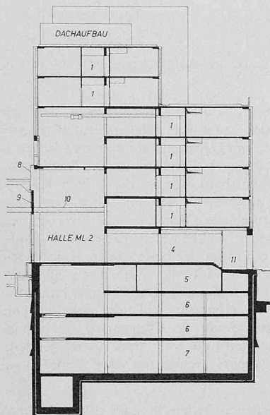
Bild 6. Querschnitt 1:600. Bezeichnungen:
