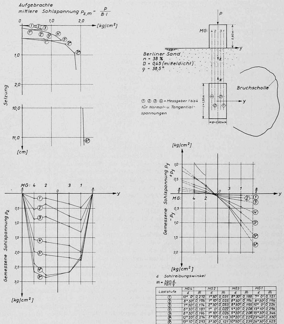
Bild 13. Last-Setzungsdiagramm eines bis zum Grundbruch belasteten Fundaments ( t = 0 , F = 0,6 \text{ m} \times 1,2 \text{ m} ) und dabei gemessene Normalspannungen und Tangentialspannungen in der Sohlfuge
