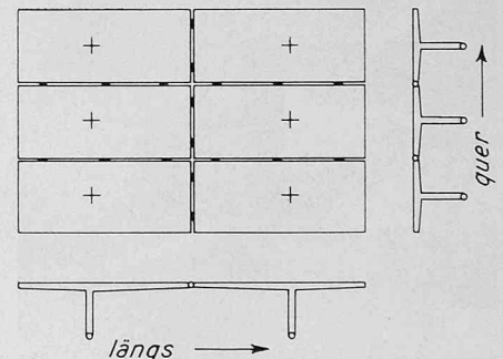
Bild 15. Statisches System
