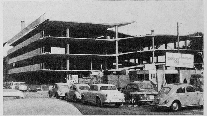
Bild 4. Ansicht des fertig montierten Parkhauses von der Stirnseite mit teilweise montiertem Gelände, Treppenhaus noch nicht montiert
