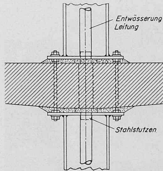
Bild 9b. Querschnitt durch die Verbindung Platte/Stütze
