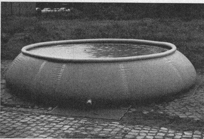
Bild 2. Offener EXCALOR-Faltpfand aus Neoprene/Hypalon-beschichtetem Polyestergewebe (Trevira), geeignet für Wasserspeicherung; Fassungsvermögen 10000 l.
