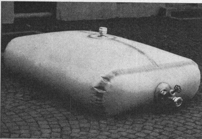
Bild 1. Geschlossener EXCALOR-Faltpfand aus Perbunan-beschichtetem Polyestergewebe (Trevira) für Wasser, Öl oder Chemikalien; Fassungsvermögen 1000 l.
