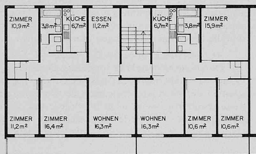
5-Zimmerwohnung, 103,5 m 2
