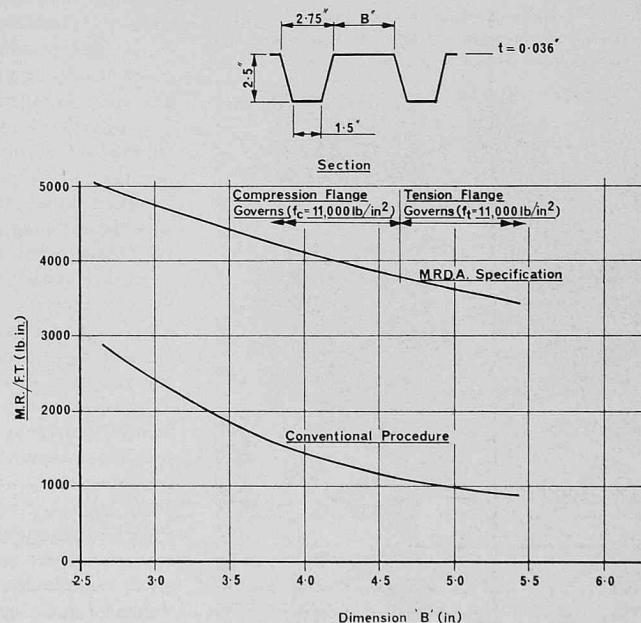
Bild 5 (rechts). Vergleich der Widerstandsmomente von Aluminiumblechtafeln bei konventioneller Berechnungsmethode und bei reduzierter Druckplattenbreite nach einer Formel auf Grund von Versuchswerten der «Metal Roof Deck Association» (Design and Technical Requirements for Light-Gauge Metal Roof Decks, October 1965):
