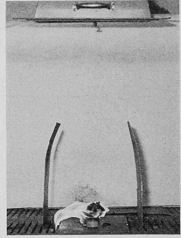
Bild 5a (links). Flammenbewegung bei Luftströmung von unten nach oben (Modellversuch)
