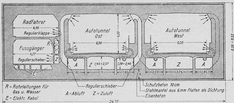
Bild 6. Querschnitt durch den Maastunnel in Rotterdam [16], 1:250
