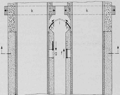
Bild 7. Vorschlag für die Gestaltung eines Kraftfahrzeugtunnels mit Sicherheitsvorrichtungen im Brandfall a Fahrraum, b Frischluftkanal, c Abluftkanal, d Fussgängertunnel, e Frischluftkanal zu d, f geschlossene Tür, g geöffnete Tür, h Seitentüren, i verschliessbares Portal, k Fussgängerunterführungen
