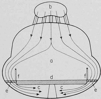
Bild 4. Vorschlag für die Querschnittsgestaltung eines querbelüfteten Kraftfahrzeugtunnels mit Lüftungsrichtung von oben nach unten. a Fahrraum, b Frischluftkanal, c Abluftkanal, d Fahrbahn mit leicht gewölbter Decke, e Laufgitter, f Geländer
