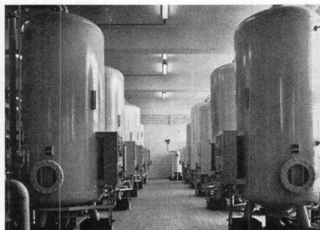
Kesselspeisewasser
