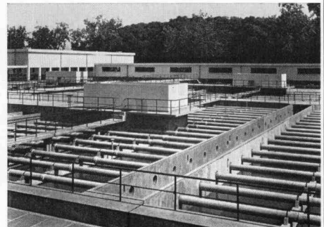
«PULSATOR» für Wasseraufbereitung
