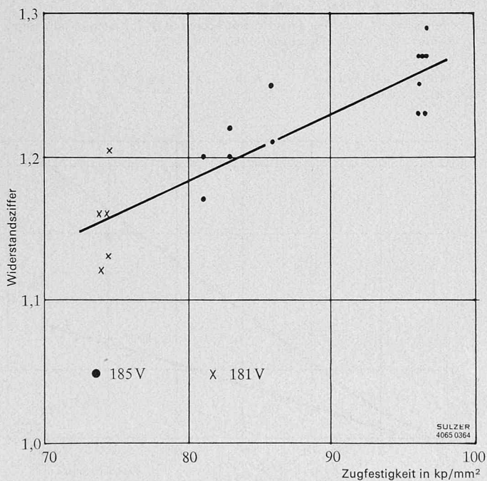
Bild 17. Widerstandsnummer von Stahlguss 181 V bzw. 185 V in Abhängigkeit von der Zugfestigkeit
