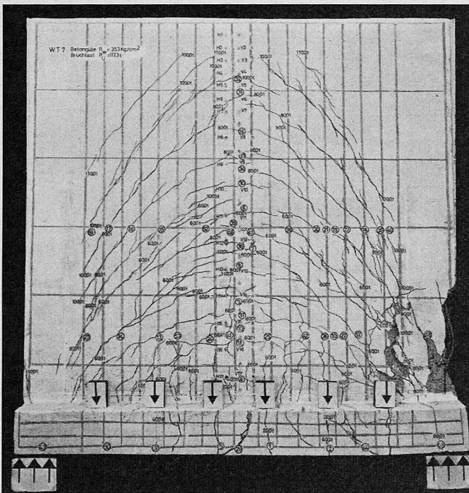
Bild 9. Wandartiger Träger WT 7 ( \mu = 0,268\% ) nach dem Bruch bei P_U = 117,3\text{ t} . Bruchursache: Versagen des Betons auf schiefer Druck in der Kämpferzone der Gewölbe
