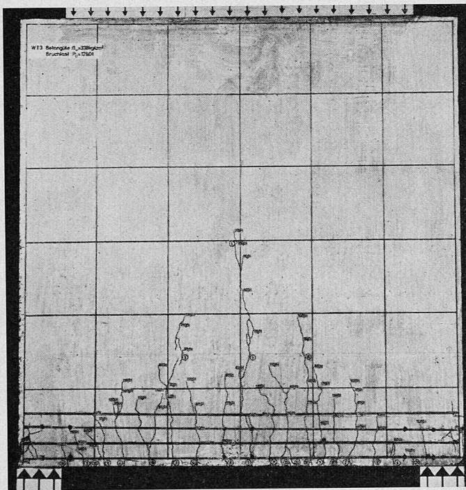
Bild 5. Wandartiger Träger WT 3 ( \mu = 0,268 \% ) nach dem Bruch bei P_U = 129,0 \text{ t} . Bruchursache: Versagen der Auflagerzonen bei p_a = 403 \text{ kp/cm}^2 = 1,33 \beta_p
