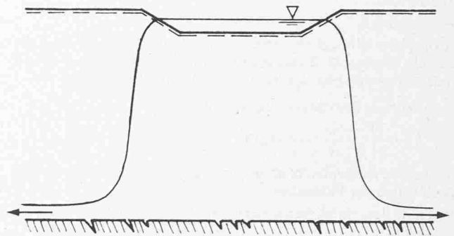
Bild 16. Freie Infiltration
