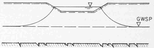
Bild 15. Rückgestaute Infiltration
