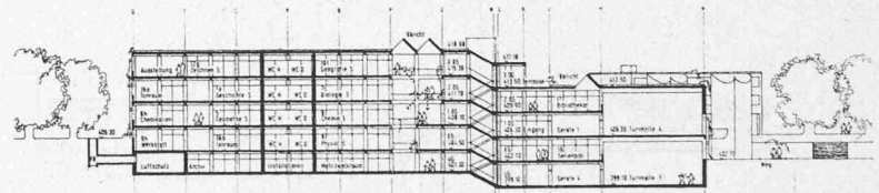
Längsschnitt Unterrichtstrakt/Turnhallentrakt 1:1200
