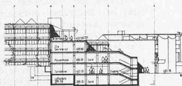
Schnitt Treppenhaus/Turnhallentrakt 1:1200
