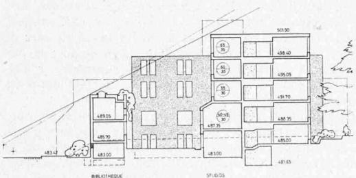
Schnitt Bibliothek-Studios 1:750
