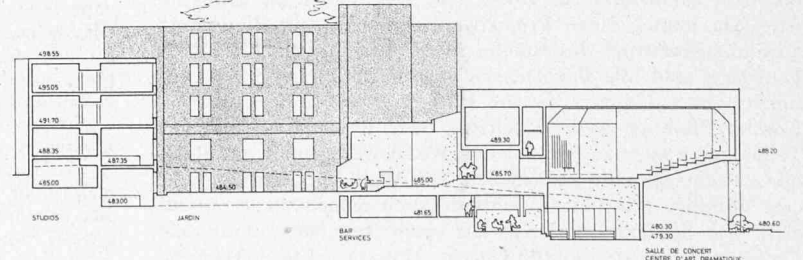
Schnitt Studios-Gartenhof-Konzertsaal 1:750
