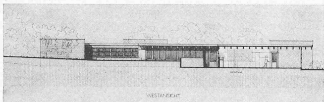
Westansicht
