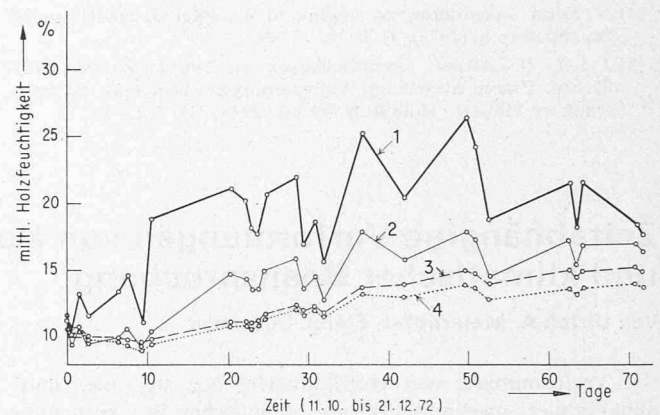
Bild 7. Zeitlicher Verlauf der Holzfeuchte von Tüferr Brettern auf einer Südwestfassade in Abhängigkeit von der Feuchtigkeitsschutzwirkung der Oberflächenbehandlung. Angaben für Fichtenholz: 1 unbehandelt, 2 mit rel. durchlässigem Imprägnieranstrich, 3 mit rel. undurchlässigem Imprägnieranstrich, 4 mit Kunstharzfarbanstrich
