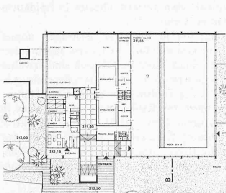
Grundriss Hallenbad 1:900
