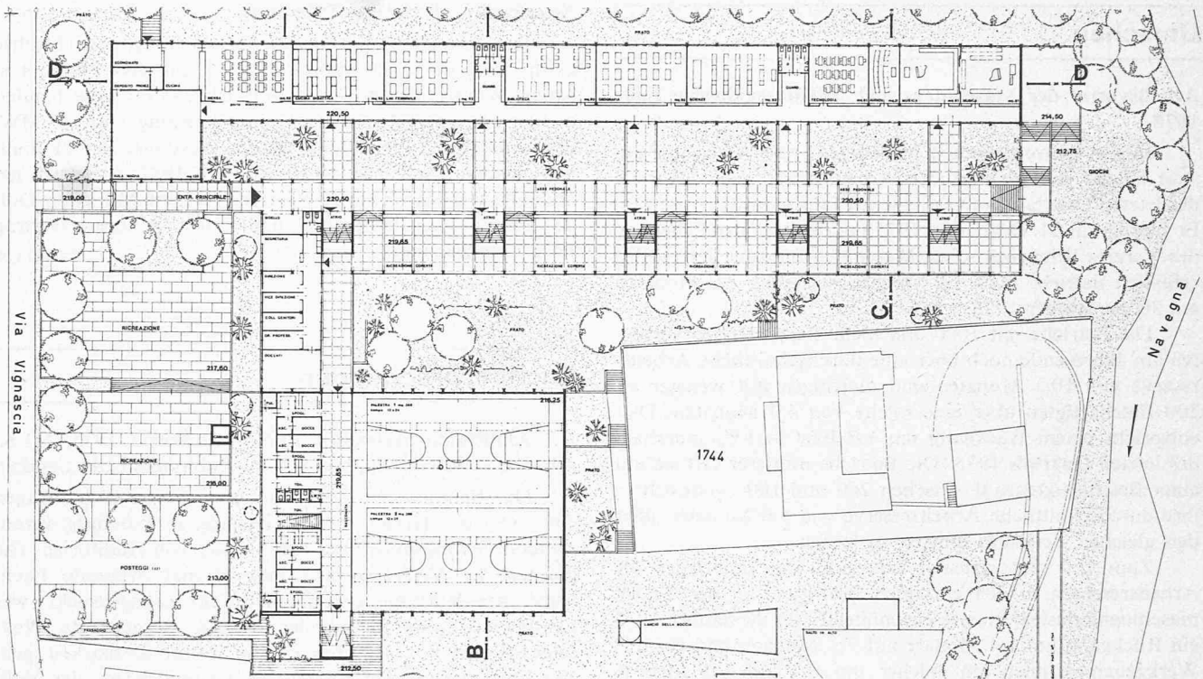
Grundriss Erdgeschoss 1:900
