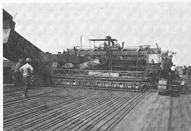
Bild 3. Die Betonverteilmaschine übernimmt Beton vom Zufuhrfahrzeug. Über ein Gummitransportband wird der Beton der Verteilmaschine in der Mitte der zukünftigen Strasse geführt. Die Verteilmaschine ist durch eine Vorrichtung ergänzt, welche dem Beton automatisch und kontinuierlich den Armierungsstahl zuführt
