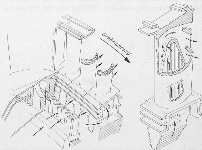
Bild 6. Kühlung der Hochdruckturbinenschaufeln. Links: Der Luftstrom wird durch Leitschaufeln beschleunigt und in die Drehrichtung der Turbine umgelenkt. Rechts: Die Kühlluft strömt mit hoher Geschwindigkeit im Schaufelinneren gegen die Eintrittskante (Prallkühlung) und tritt durch Schlitze an der Austrittskante hinaus
