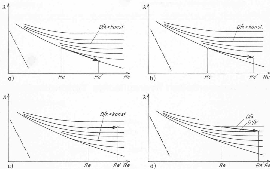
Bild 3. Veranschaulichung der Aufwertungstendenz anhand der schematisch dargestellten Widerstandsgesetze von Prandtl-Colbrook für technisch rauhe Rohre
